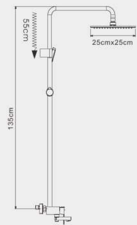
F2434 Душевая система излив является переключателем на лейку белый/хром ( в комплекте к смесителям идут 6 цветных накладок на ручку )
