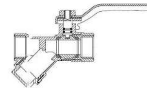
FR201 Кран ручка
