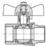
G213 Кран бабочка
